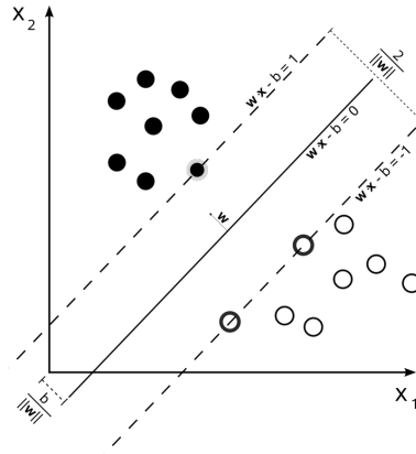
Fig. 2. 2 hyperplanes
