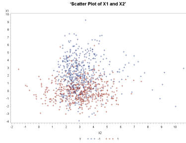
Fig. 3. 2 hyperplanes
